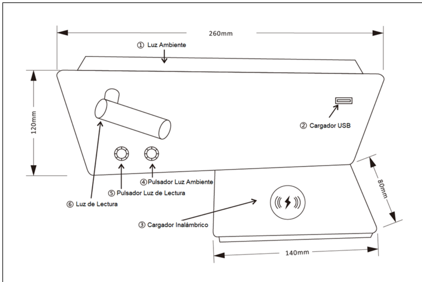
1. Cotas de la pieza
